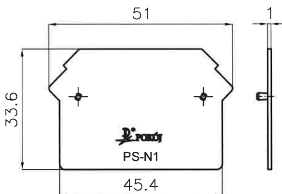
Płytki skrajna PS-N1
