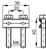
Zacisk taśmowy
