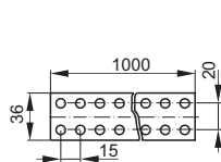
Taśma uziemiająca
