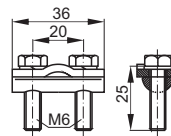
Zacisk montażowy
